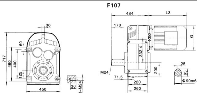
FA107/FAF107/FAZ107空心轴
