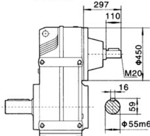
FD127
