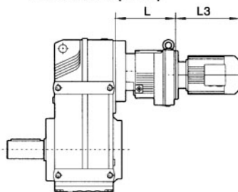
F..127R77(R87)
