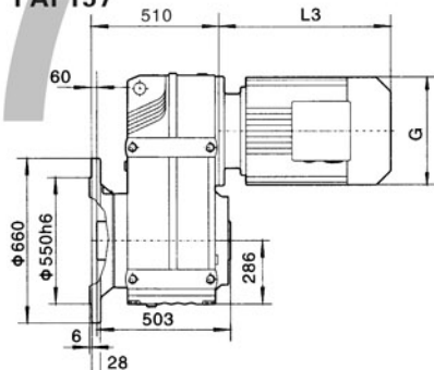
FAF157
